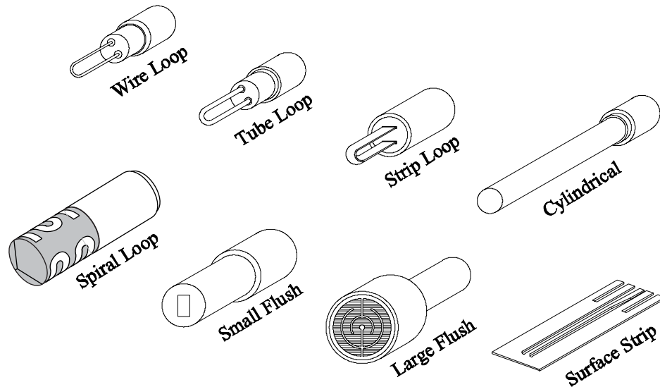
Figura 3. Elementos Sensores
