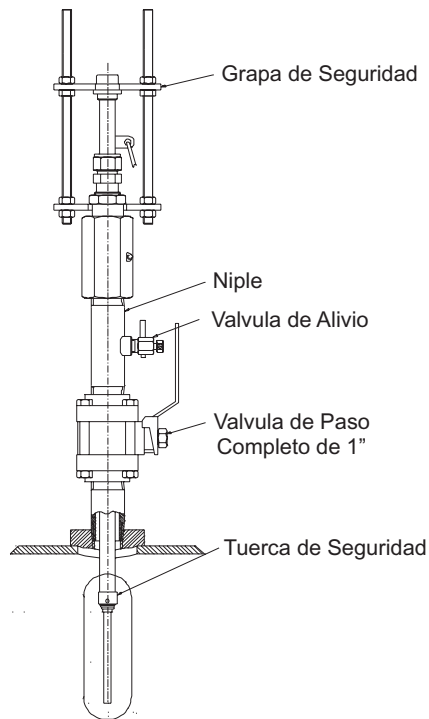
Probeta Retráctil
