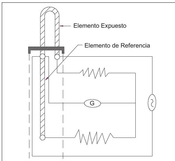
Fig. 1 Probeta / Instrumento
